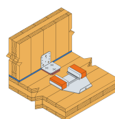
ABAI-asennus MOABAI-asennustyökalulla.
