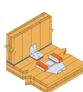
ABAI-asennus MOABAI-asennustyökalulla.
