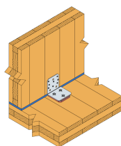
ABAI-asennus SDS-ruuveilla
