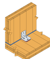
ABAI-asennus SDS-ruuveilla
