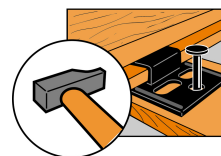
CLIP-kiinnikkeen kiinnitys nauloilla
