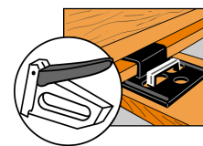
CLIP-kiinnikkeen kiinnitys niiteillä
