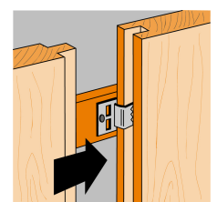
Kiinnike kiinnitetään ponttiin ja alustaan ennen seuraavan paneelin asentamista
