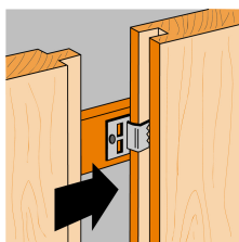
Kiinnike kiinnitetään ponttiin ja alustaan ennen seuraavan paneelin asentamista
