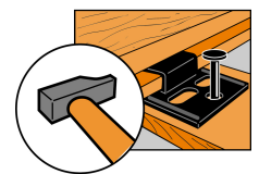
CLIP-kiinnikkeen kiinnitys nauloilla
