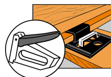
CLIP-kiinnikkeen kiinnitys niiteillä
