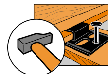
CLIP-kiinnikkeen kiinnitys nauloilla
