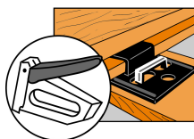
CLIP-kiinnikkeen kiinnitys niiteillä
